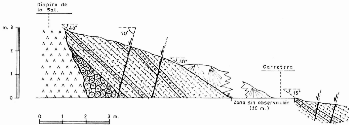
Fig. 16.—Corte neotectónico en el paraje del Faldar.
