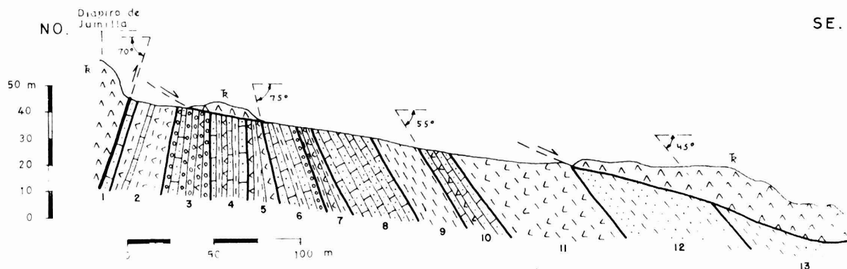
Fig. 11.—Corte neotectónico en la Rambla de los Gargantones. Tr = Triás. 1 al 13 Andaluciese-Messiniense.
