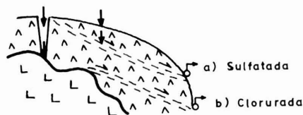
Fig. 15.—Esquema sobre los diferentes tipos de manantiales en el diapiro de Pinoso.
