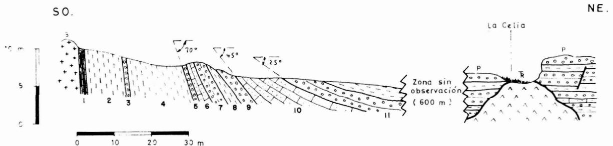
Fig. 9.—Corte neotectónico en las proximidades de La Celia. \beta =Rocas volcánicas. T_R = Triás. I al II y P=Plioceno (I. Metasomatismo de contacto)
