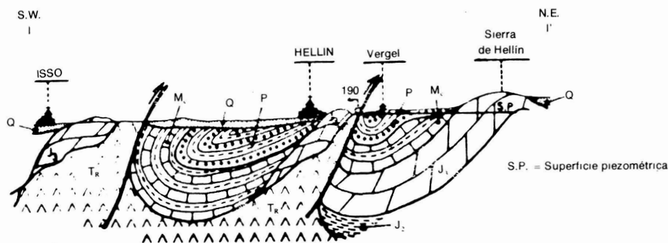
Fig. 3.—Esquema hidrogeológico de la fuente de Hellín. T R = Trías. J 2 = Lías medio. J 3 = Dogger. M c = «Pontiense». P = Plioceno. Q = Cuaternario.
