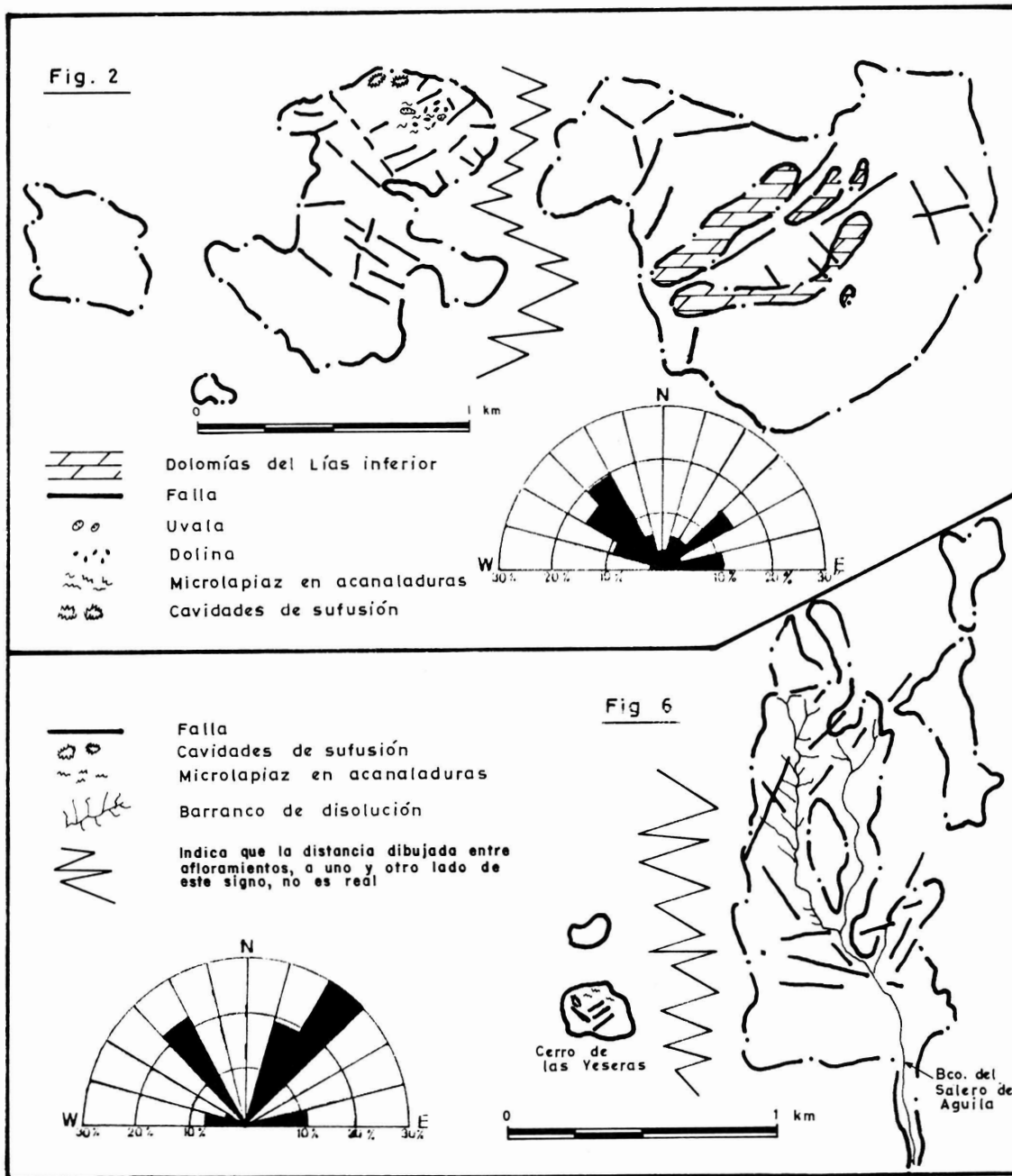
Fig. 6.—Mapa morfoestructural del diapiro de Ontur.
