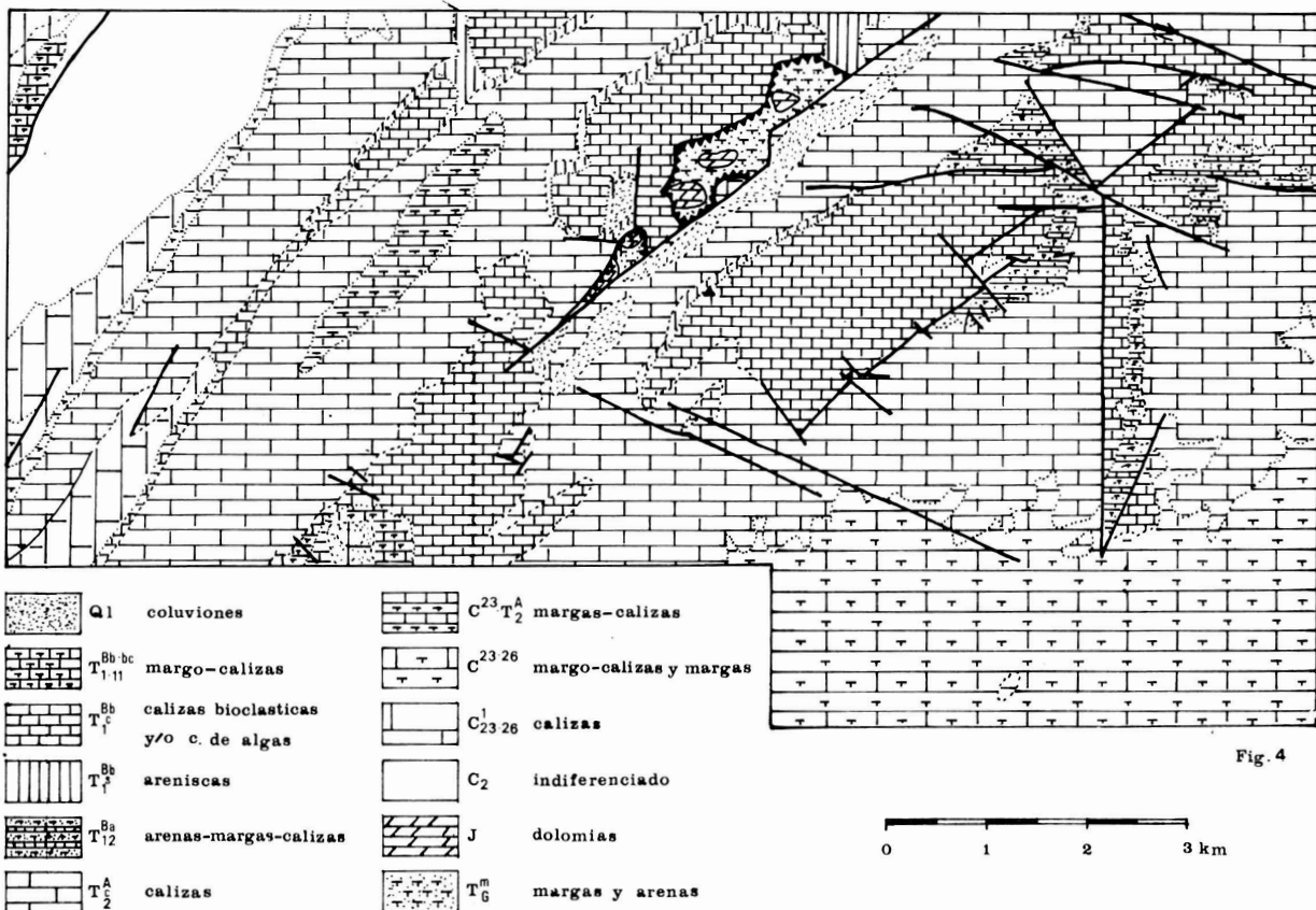
ESQUEMA LITOLOGICO
