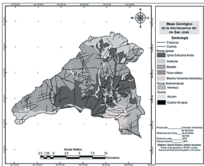
FIGURA 2: Componentes litológicos de la microcuenca
