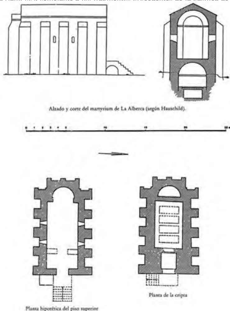
Figura 3. Reconstrucciones probables del Martyrium de La Alberca según Hauschild. (Molina Gómez, 2004: 13).
