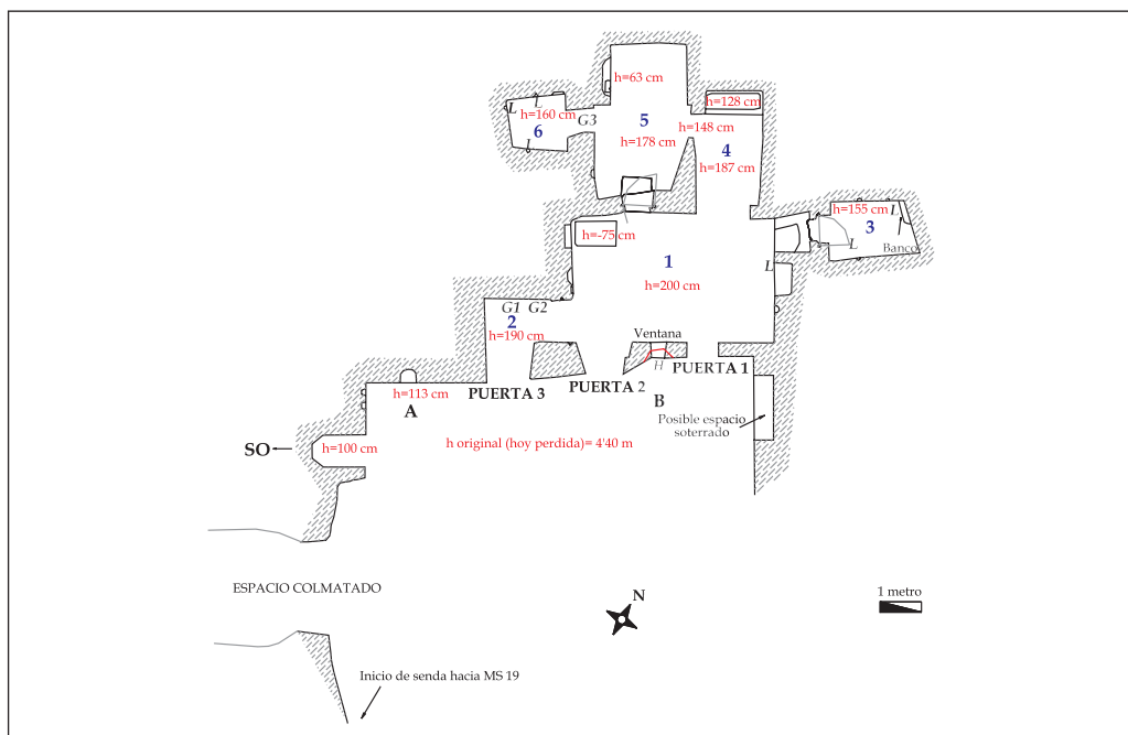
FIGURA 156. Planta de MS/17
