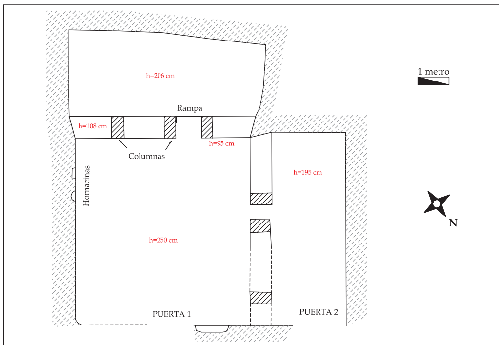
FIGURA 126. Planta de MS/1
