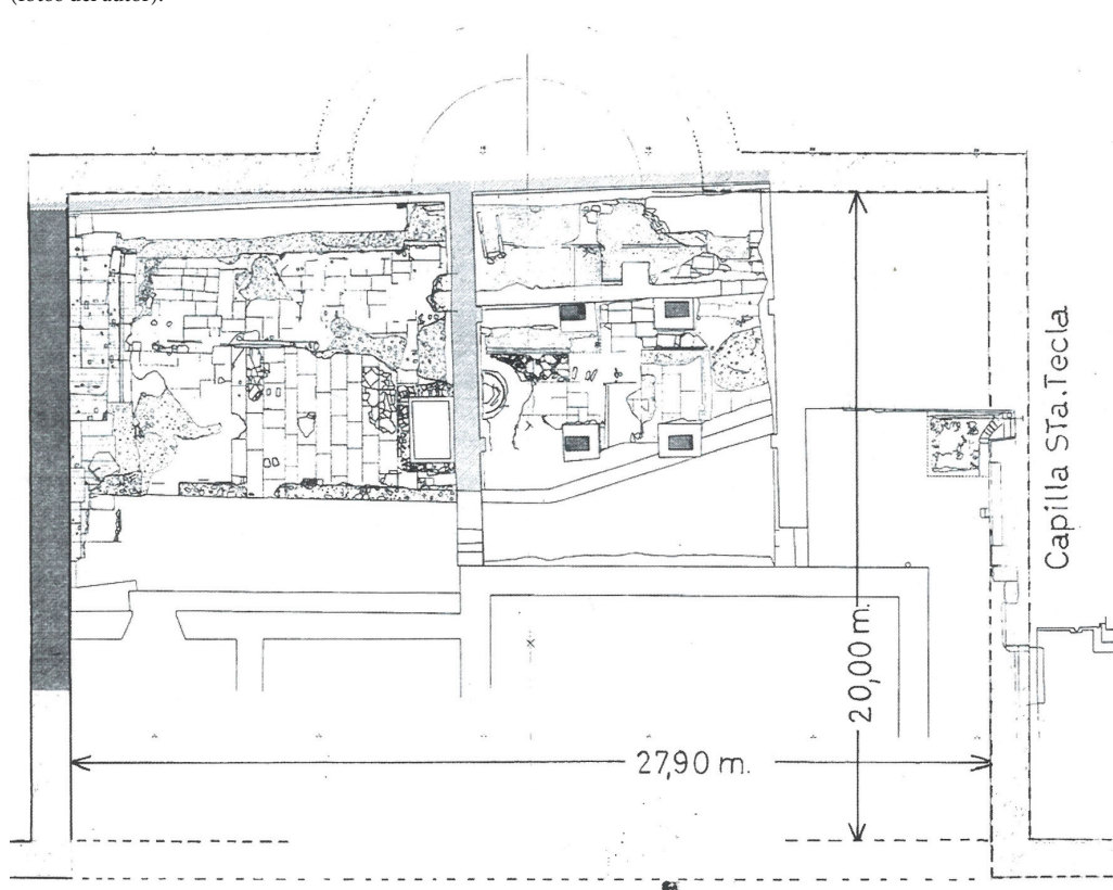
Figura 4. Arriba: Planimetría de los restos conservados de la sala-aula axial (Hauschild 2009, fig. 15).
