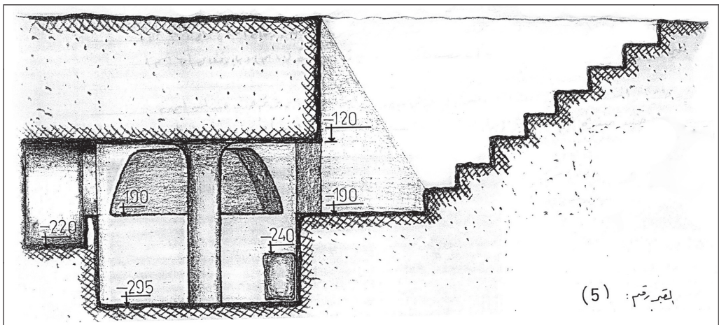
FIGURA 4. Croquis de un hipogeo con columna central excavado por el Museo de Deir ez-Zor. Escala 1/25. Omar al-Talfah y Taif al-Yalabi, 2003.
