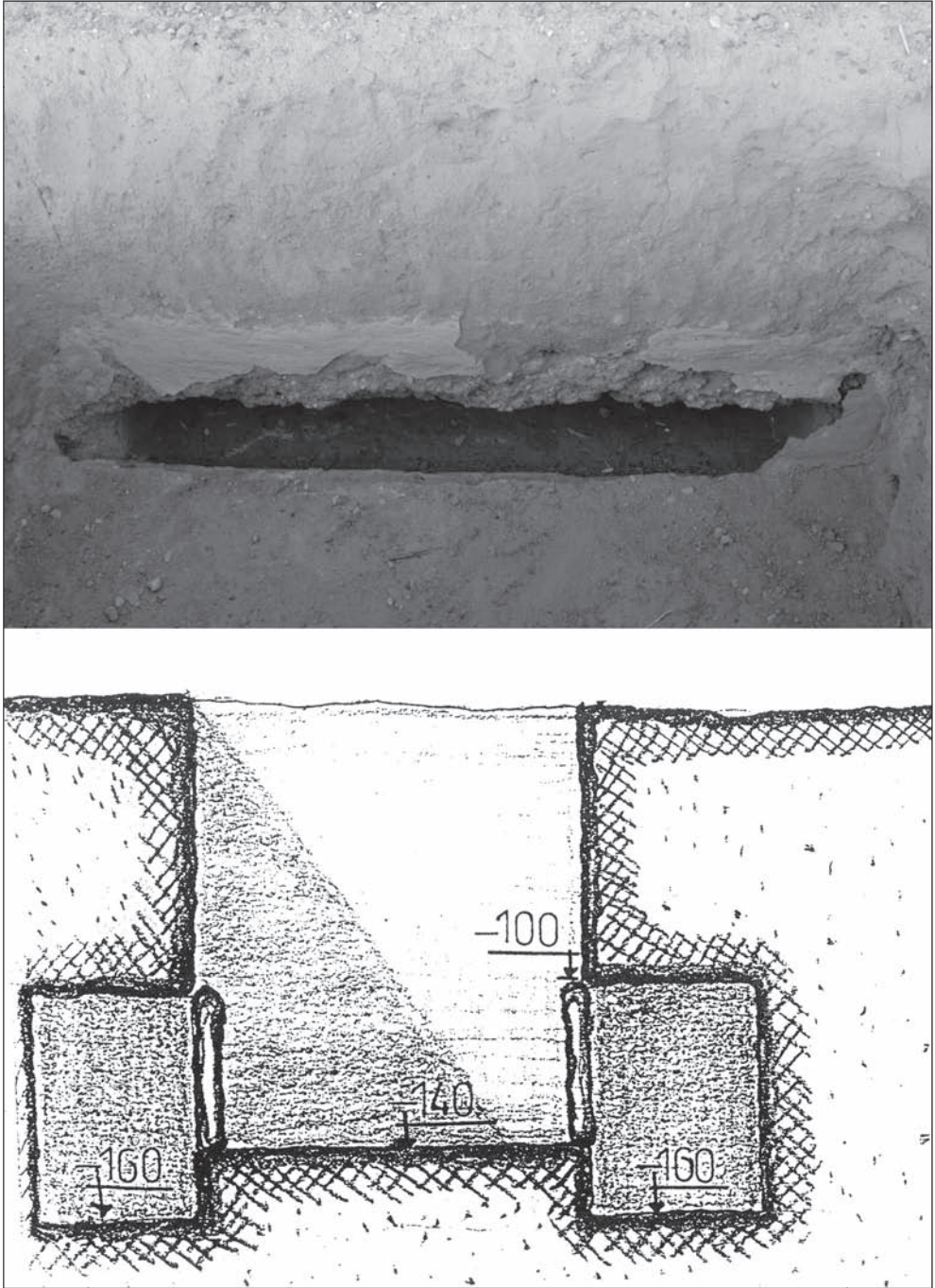
FIGURA 5. Croquis y foto de una tumba en fosa con dos nichos laterales. Escala 1/25. Omar al-Talfah y Taif al-Yalabi, 2003.
