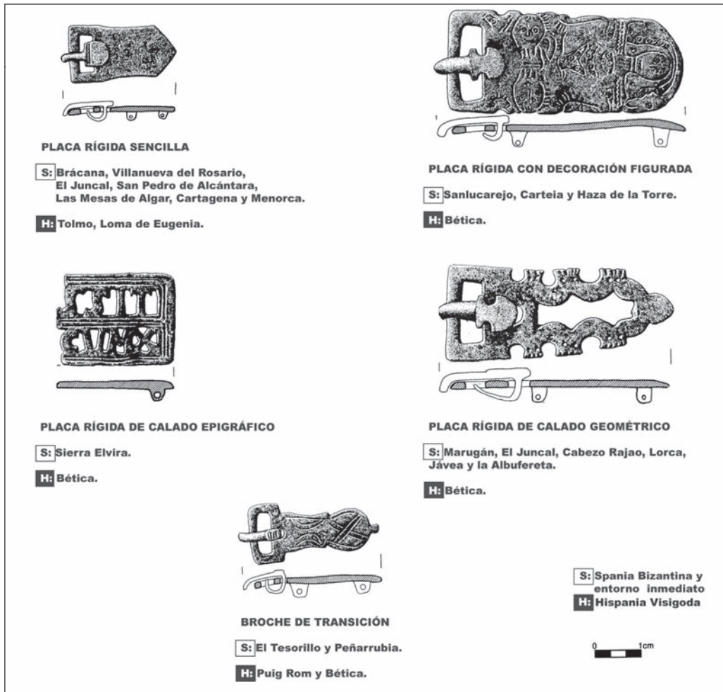
FIGURA 117: Tipos de broche de cinturón de placa rígida documentados en el Mediodía hispano (a partir de Ripoll, 1998)
