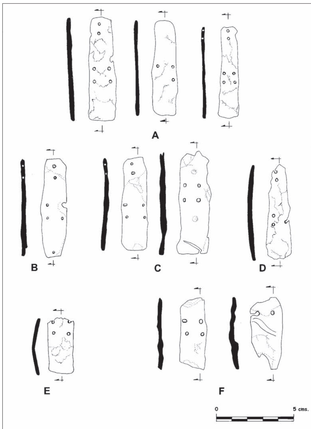
FIGURA 121: Tipos de lámina empleados en la coraza hallada en el barrio de época bizantina de Cartagena (Vizcaíno Sánchez, 2008d). Dibujo: Soledad Pérez Cuadrado
