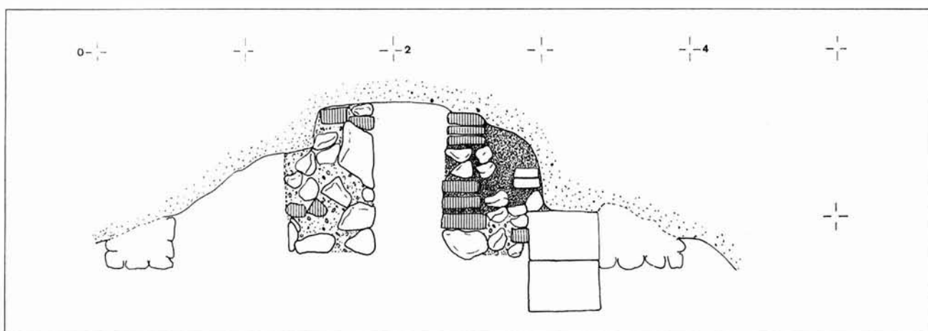
FIGURA 3.- Sección C-C'.
