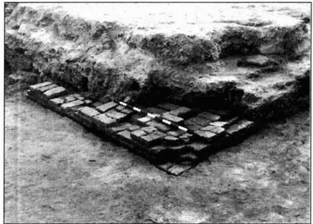
FIGURA 6. Detalle del torreón de la figura anterior. Esquina reparada mediante ladrillos.
