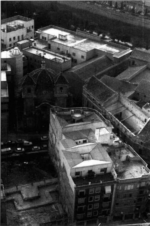
FIGURA 4. Vista de la excavación de un tramo de la muralla que separaba el alcázar de la medina. La imagen está tomada desde la torre de la catedral, antigua mezquita aljama. En el centro de la imagen, la iglesia de S. Juan de Dios; al fondo, el río Segura. En el ángulo superior izquierdo se halla el edificio de la Delegación del Gobierno, sobre el solar de la Torre de Caramajul.
