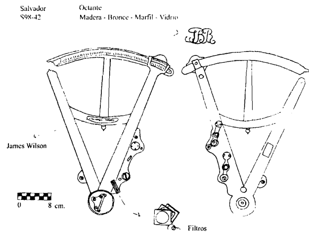
FIGURA 1. Octante encontrado en el navío «El Salvador» (1812) (dib. A. Lezama).
