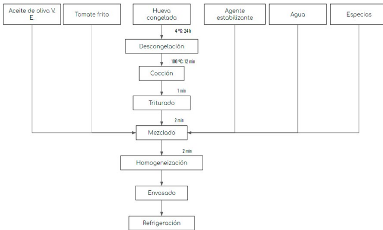
Figura 3. Diagrama de flujo paté de hueva
