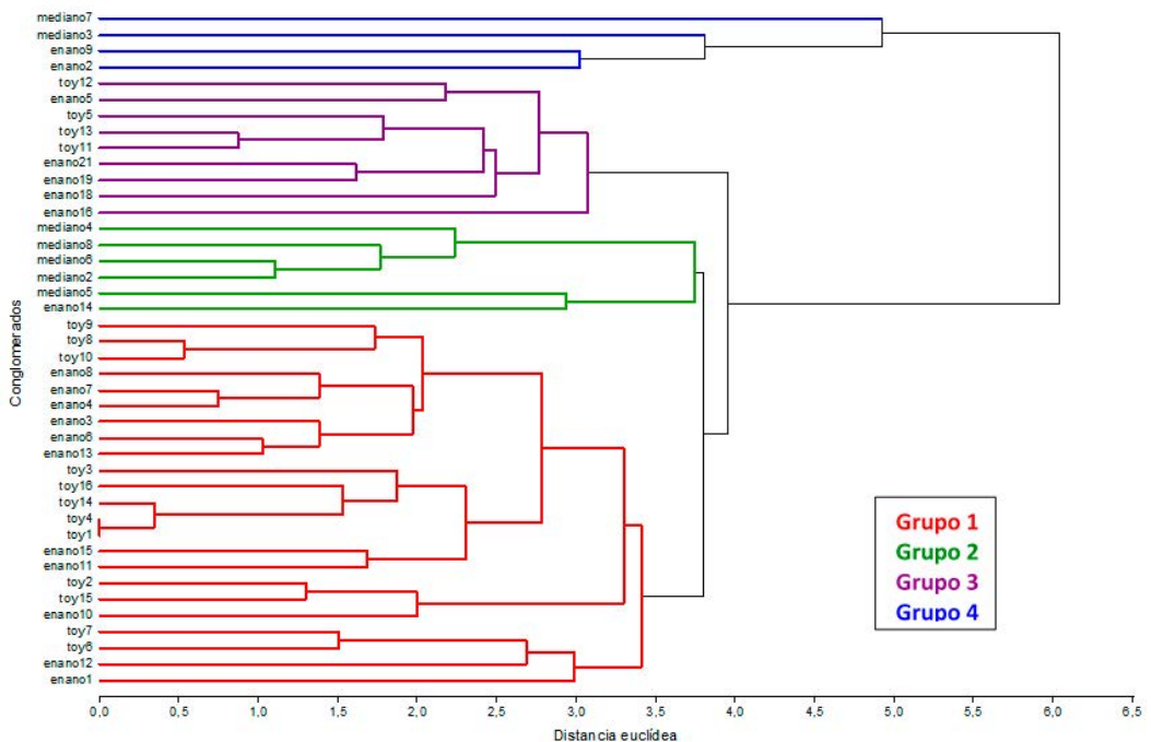
Figura 5. Dendograma construido a partir de una matriz de distancia euclídea mediante el sistema de agrupamiento por promedios simples. El análisis multivariante incluyó todas las variables, y se consideraron los Caniches con un seguimiento \leq 18 meses ( n=42 ). Se observan 4 conglomerados, identificados como grupo 1 ( n=23 ), grupo 2 ( n=6 ), grupo 3 ( n=9 ) y grupo 4 ( n=4 ).
