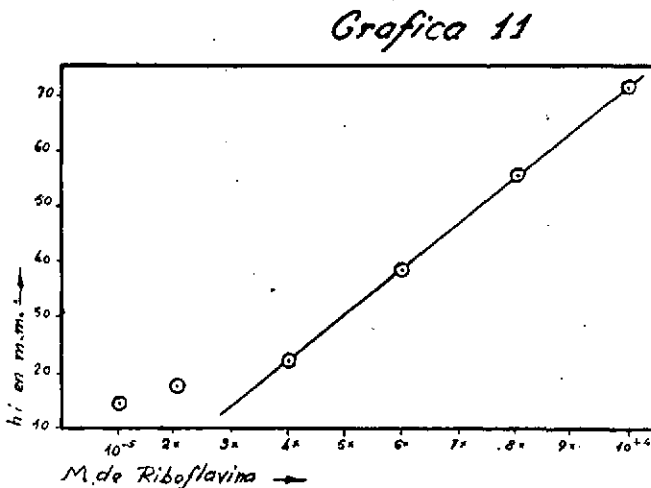
Límite cuantitativo de la onda de riboflavina en CIK 0,1 N sin regular a pH 6,00
