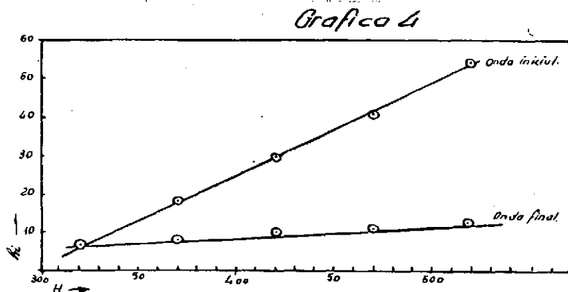
Análisis de las ondas inicial y final de la onda anódica de la tiamina en ClK 0,1 N, regulando con borato-sosa a pH 9,40
