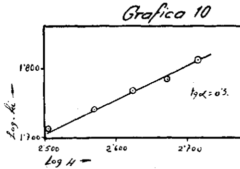
Análisis de la onda de riboflavina en CIK 0,1 N regulando con borato-sosa a pH 10,52
