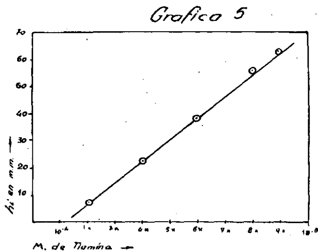
Límite cuantitativo de la onda anódica de la tiamina en ClK 0,1 N, regulado con borato-sosa a pH 9,52
