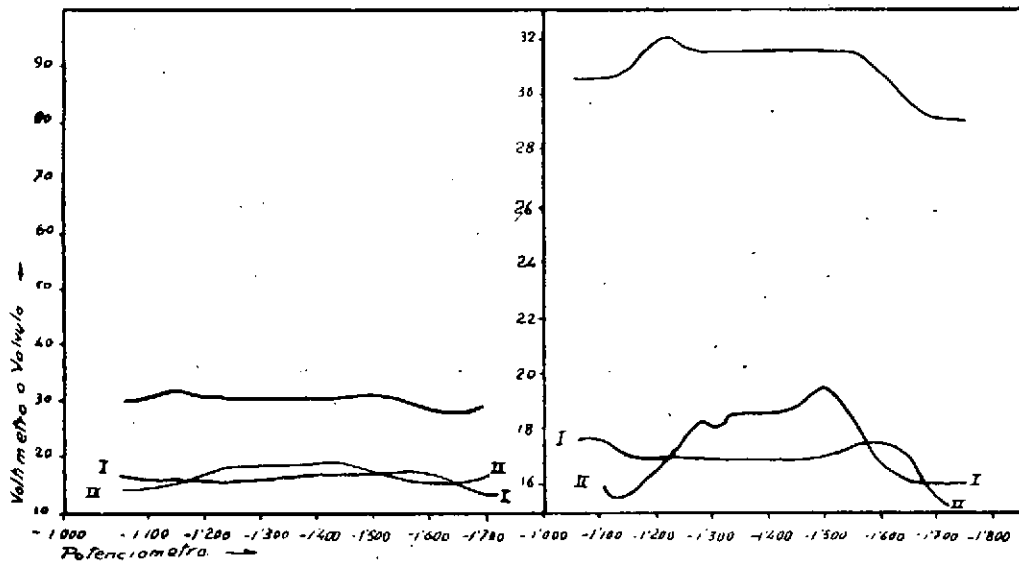
Curva de campana de la onda de ácido nicotínico en CIK 0,1 N sin regular a pH 4,12
