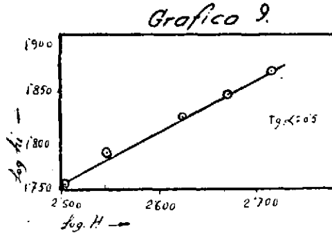
Análisis de la onda de riboflavina en CIK 0,1 N sin regular a pH 6,00
