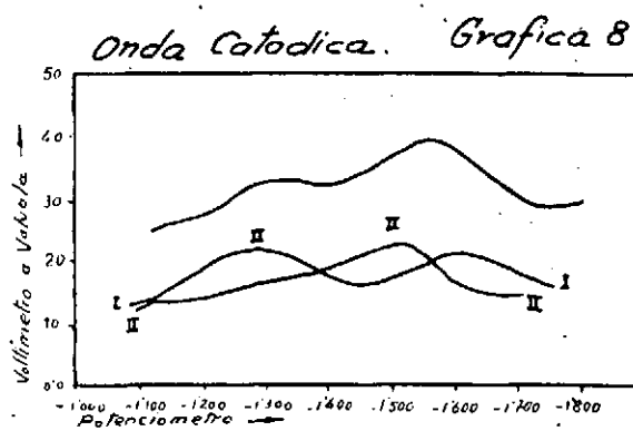
Curva de campana correspondiente a la onda catódica de la tiamina en ClK 0,1 N sin regular a pH 9,40
