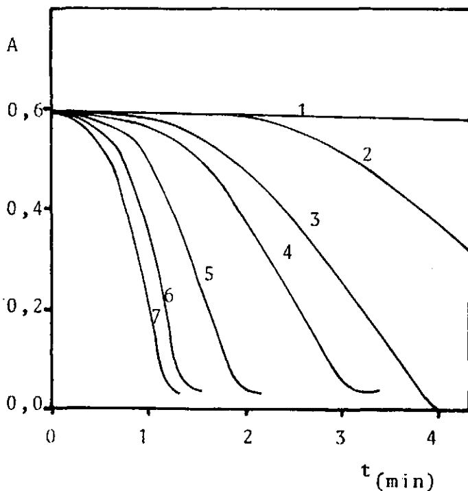
Fig. 3.—Influencia de la concentración de hipofosfito. Azul Nilo 4 \cdot 10^{-5} M; H_2SO_4 0,20 M; Pd(II) 0,10 \mu\text{g/ml} . Curva (1) sin H_2PO_2^- ; (2) 0,05 M H_2PO_2^- ; (3) 0,07 M; (4) 0,10 M; (5) 0,15 M; (6) 0,20 M; (7) 0,25 M.
