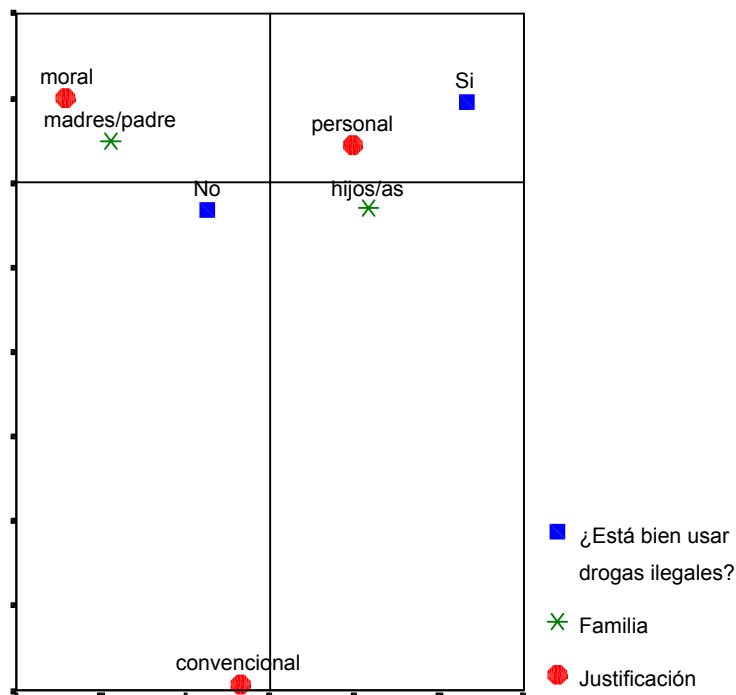
Figura 1: Análisis de correspondencias
