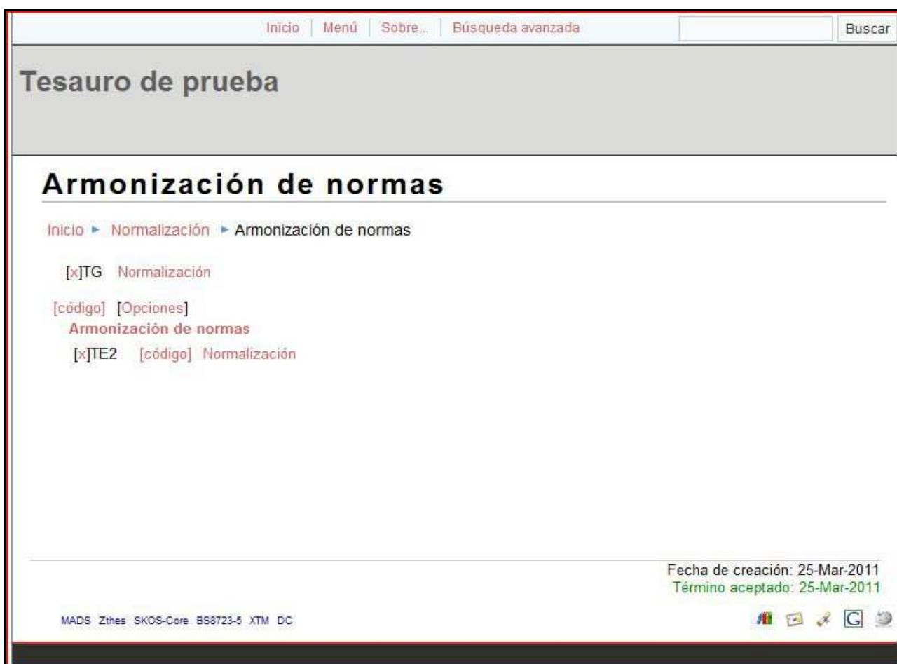
Figura 5. TemaTres.
